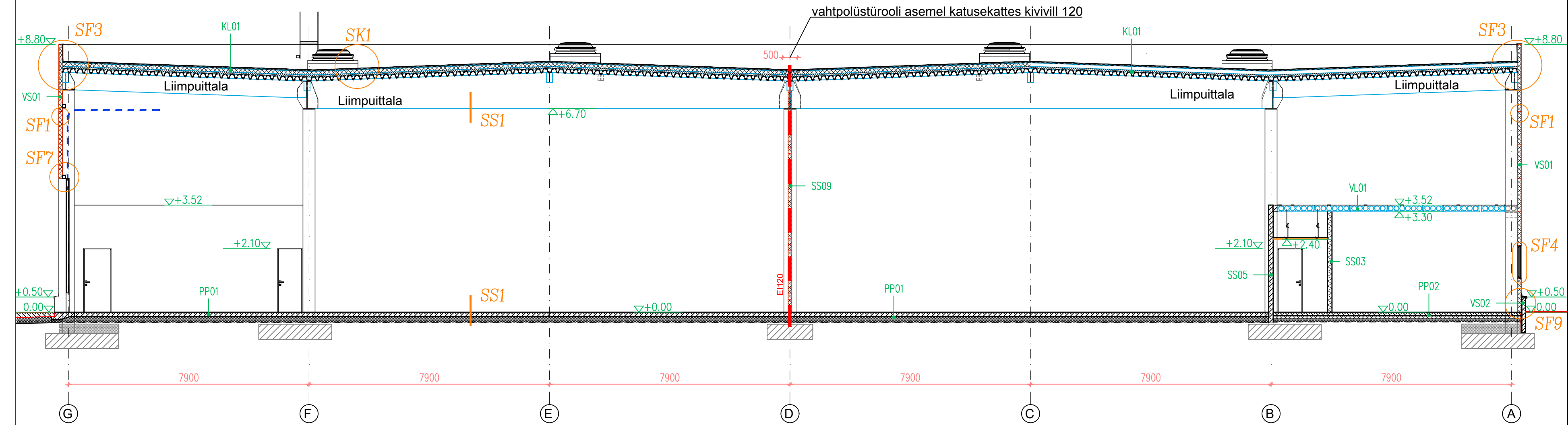
Lõige 1 - 1
